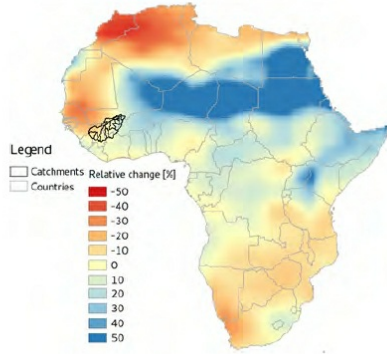
(d) NorESM
